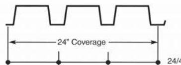
3", Type "N"
